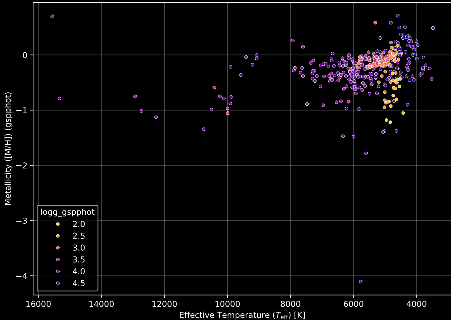
APOGEE DR17 Field: [ORIONOB1AB-B] Stellar Population Parameters (n= 385)
